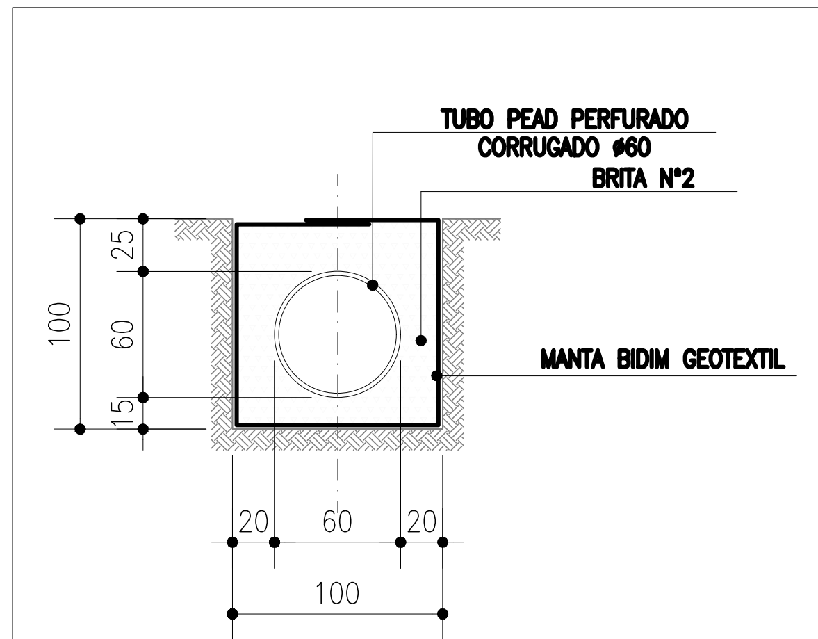
SEÇÃO TRANSVERSAL ESCALA 1:25
