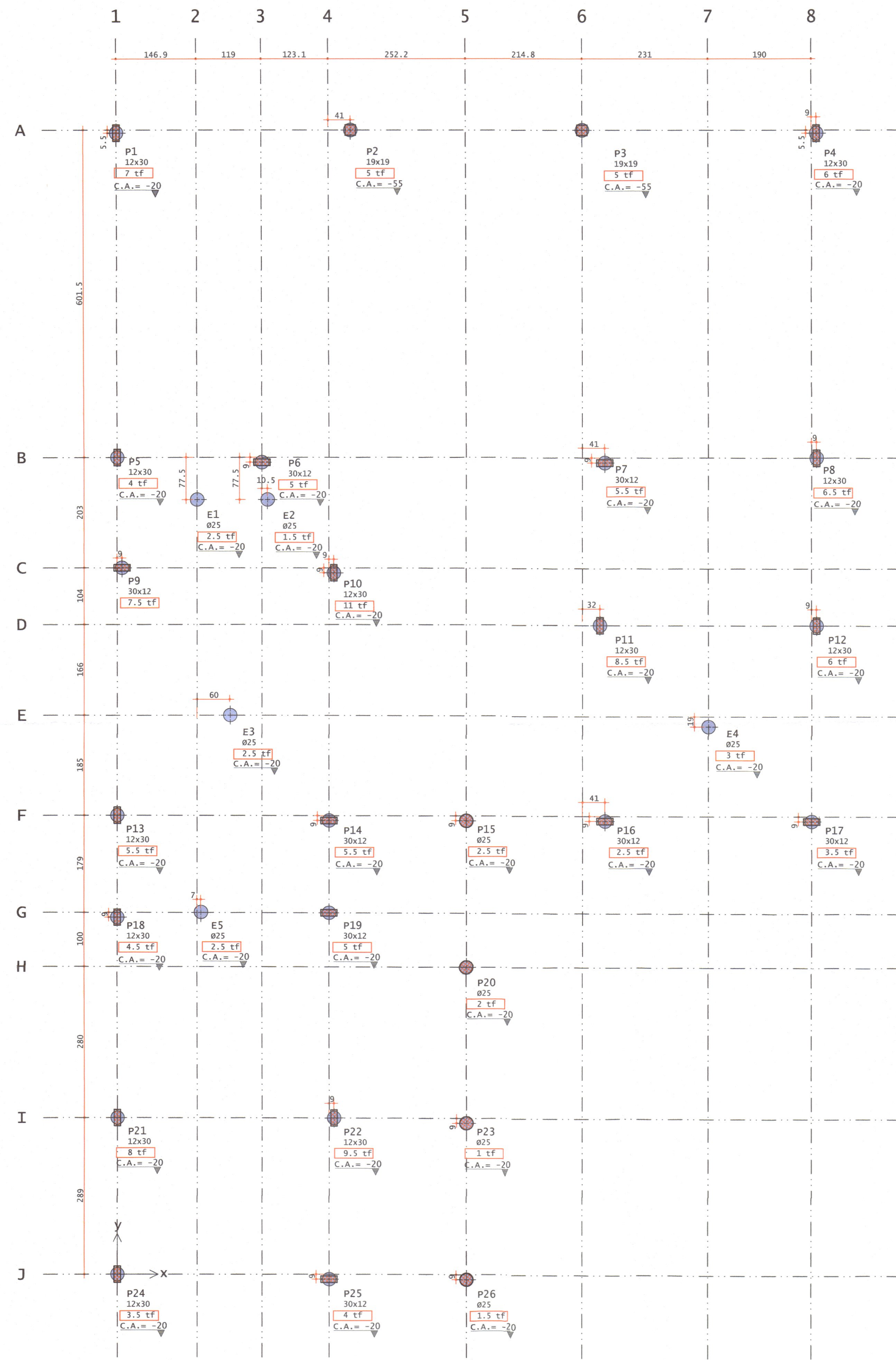
LOCAÇÃO E CARGAS DA FUNDAÇÃO ESC. 1:50
