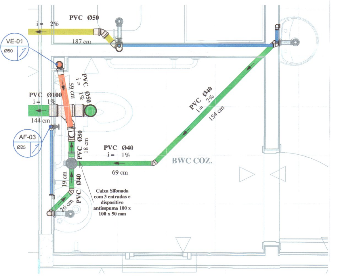
02 DET. -BWC COZ. ESCALA: 1:20
