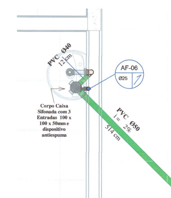
04 DET. -ATENDIMENTO ESCALA: 1:20
