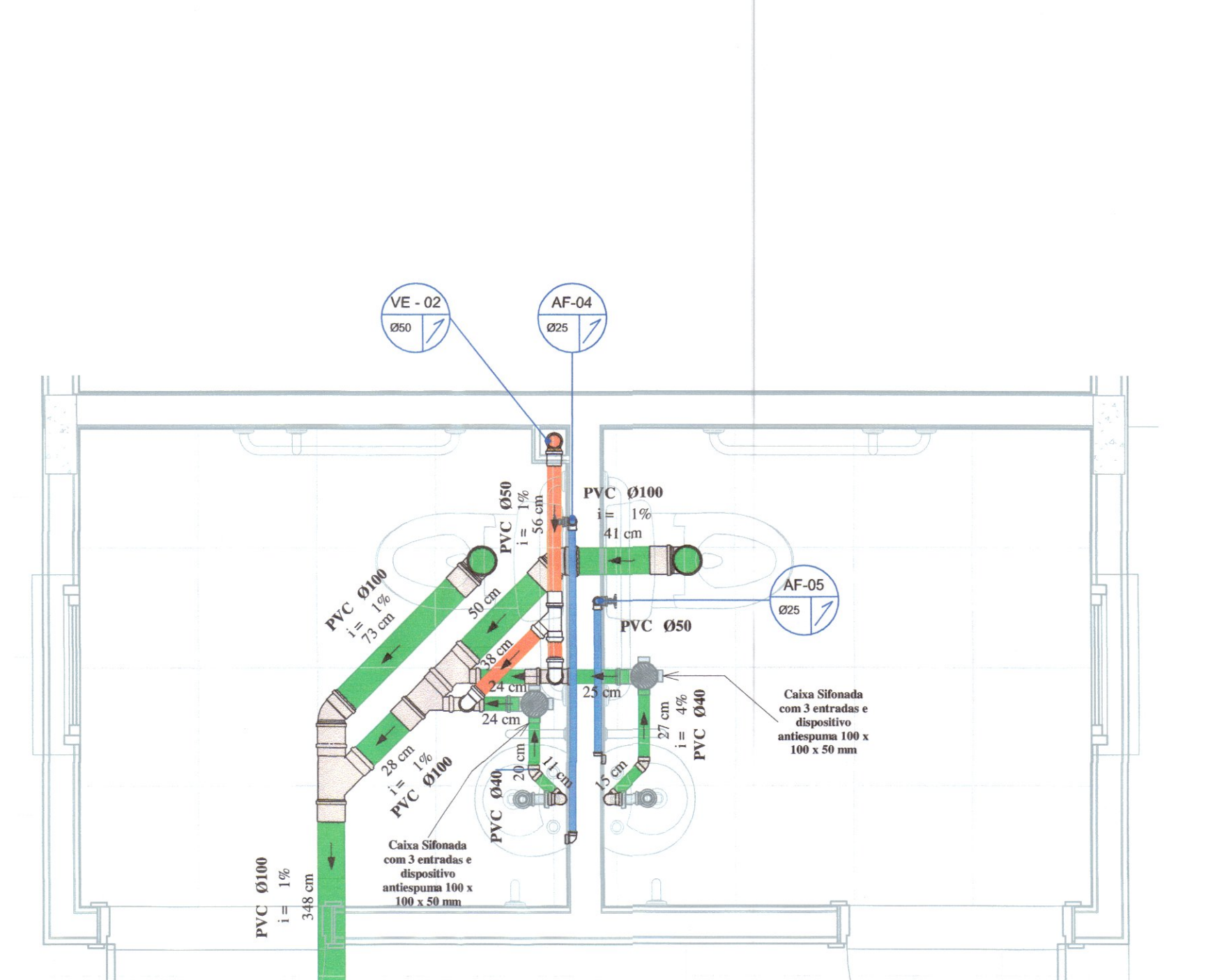
03 DET. -BWC A e B ESCALA: 1:20
