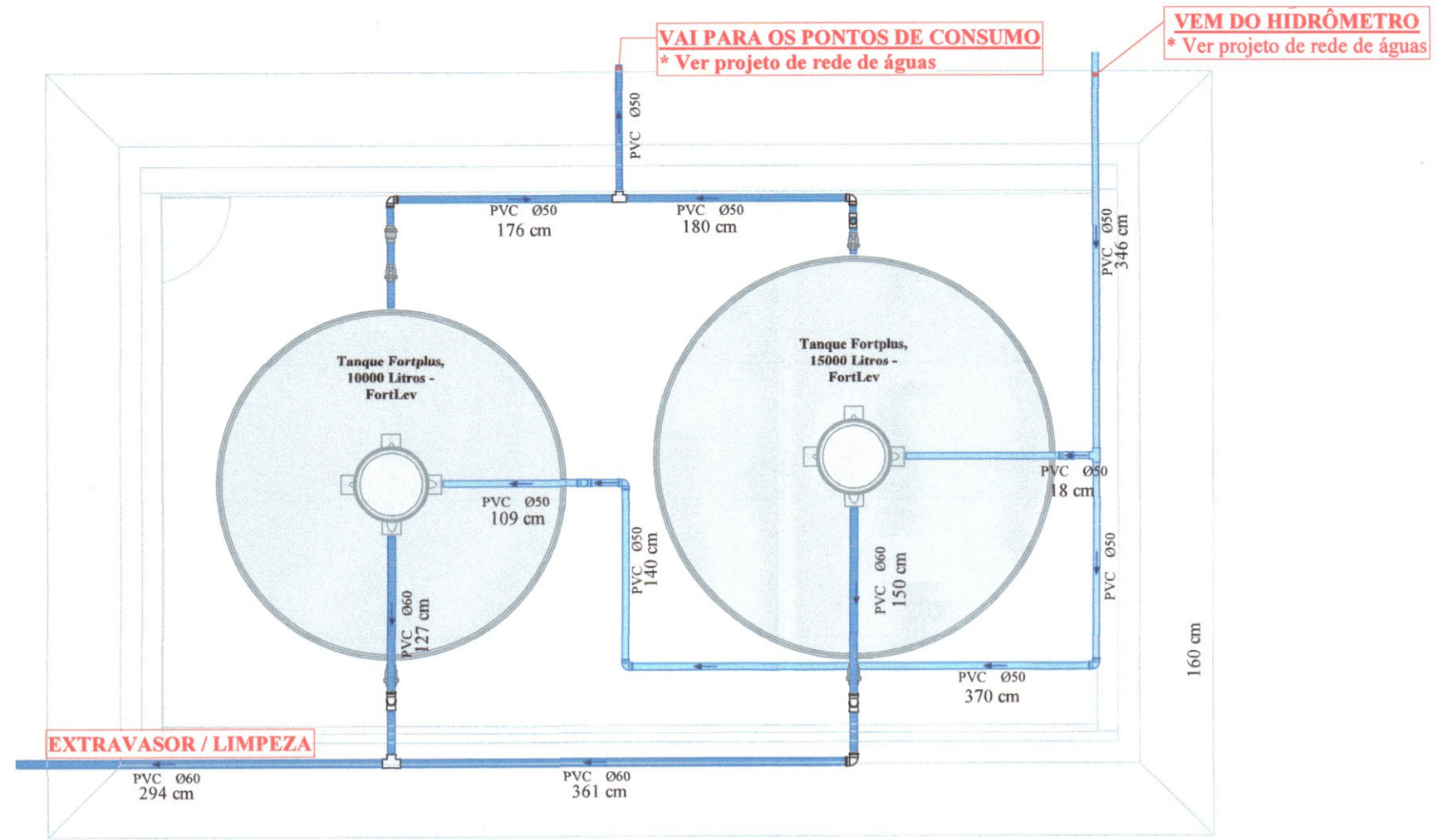
PLANTA BAIXA - TÉRREO ESCALA: 1:50
