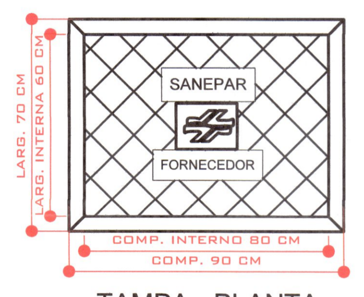
TAMPA - PLANTA
