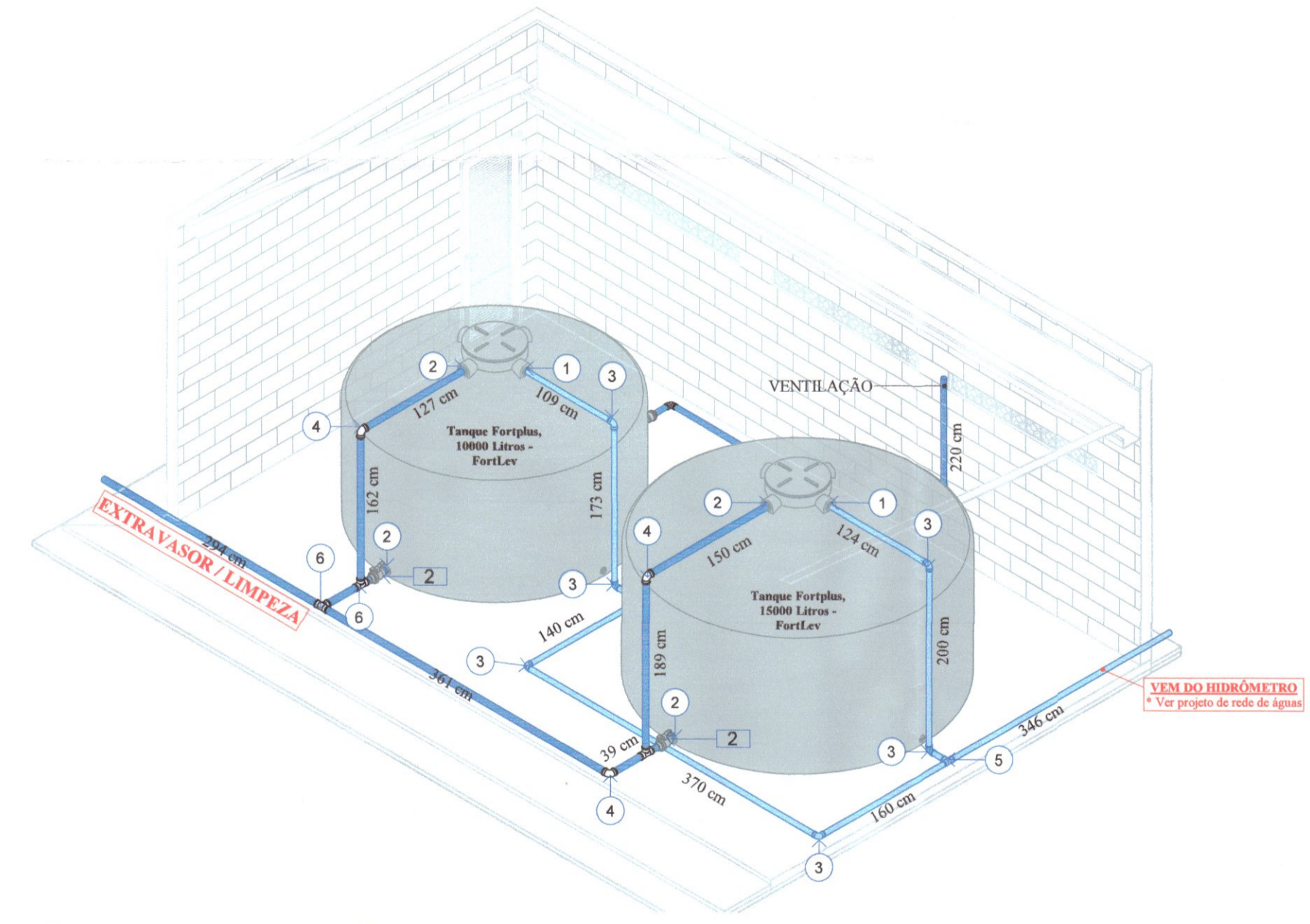
ISOMÉTRICO RESERVATÓRIOS VISTA POSTERIOR ESCALA:
